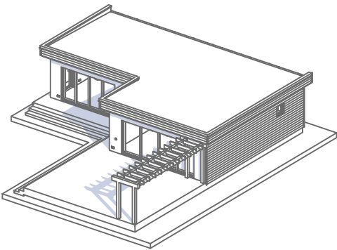
Аксонометрия крыши
